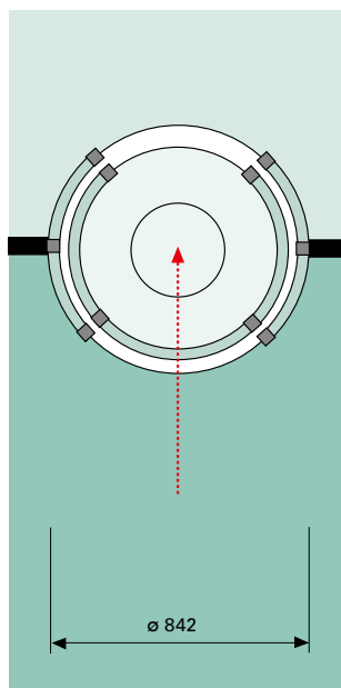
Rundschleuse Typ ZF3-1
